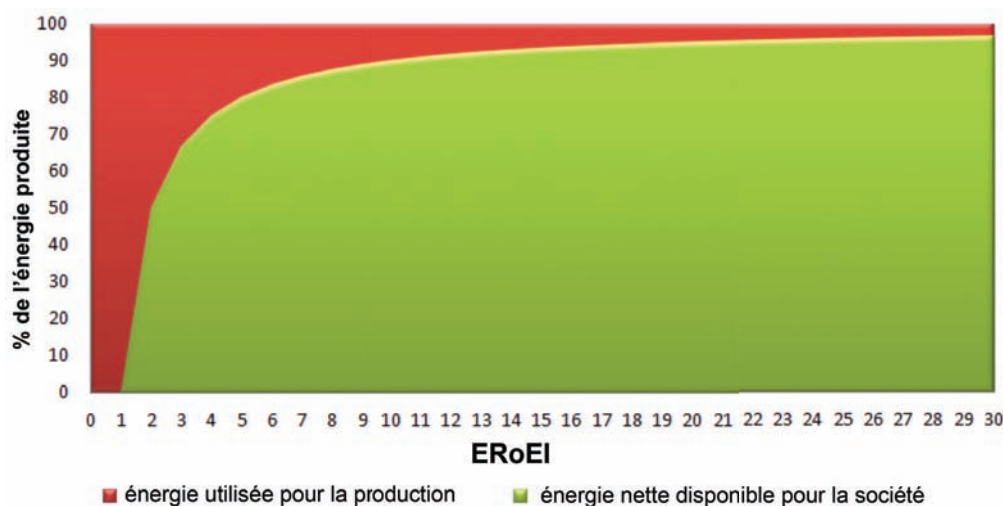
Figure 11: Evolution de l'énergie nette en fonction de l'EROEI
