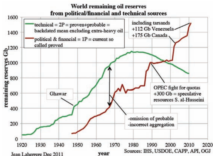
Figure 4: Réserves pétrolières mondiales restantes d'après les sources politiques, financières et techniques (Source : Jean Laherrère 4 )
