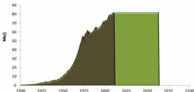
Figure 5: Futur de la production mondiale de pétrole, Ratio R/P 2012 (Données BP 2012)
