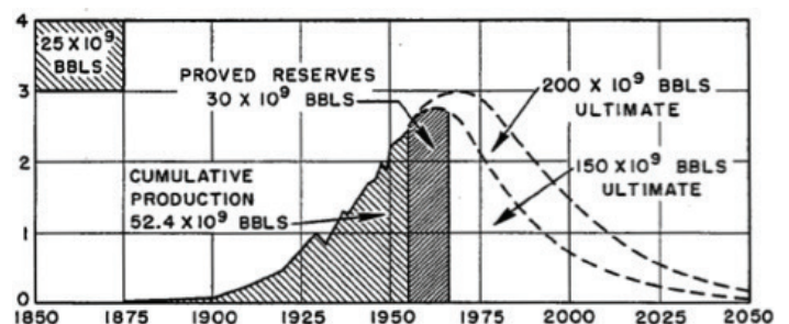
Figure 6: Modélisation de Hubbert appliquée à la production pétrolière américaine, pour 150 Gb et 200 Gb de réserves ultimes
